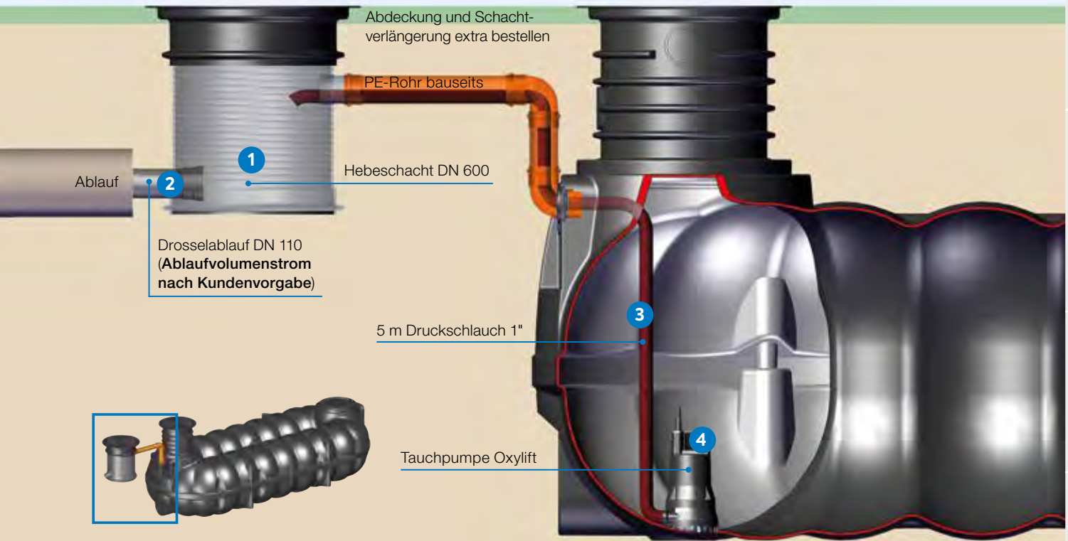
Grafikbeispiel: Retentions-Hebeschacht (mit Abdeckung begebar und Schachtverlängerung) vor dem Flachtank NEO
